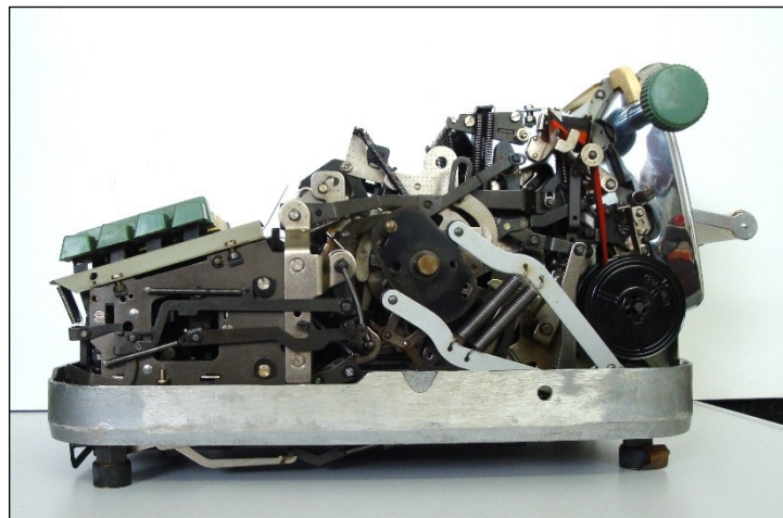
Abb. 4: Seitenansicht Modell 441-016, Gehäuse-Oberteil und Bodenwanne abgenommen.
