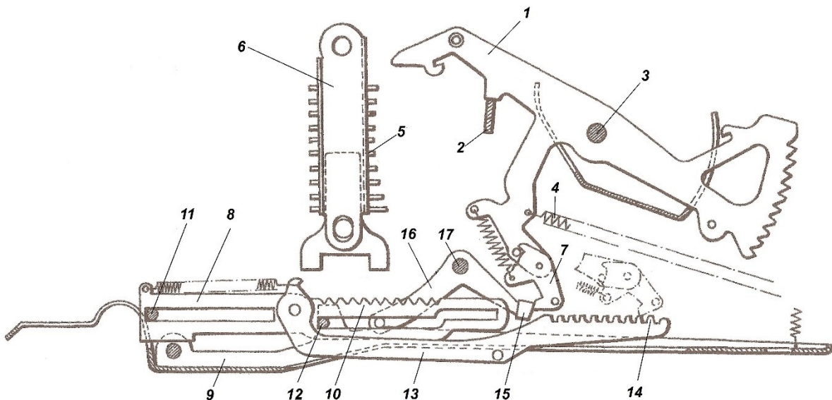
Abb. 6: Seitenansicht der Multiplikationseinrichtung
