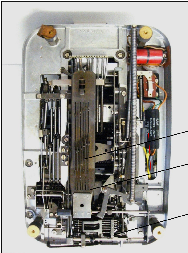
Abb. 5: Multiplikations- einrichtung;
